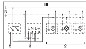
3. Ühendus käsi- või automaatujuhtimise ja jadaühendusega lülitiga
