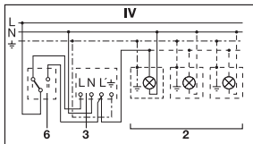
4. Priključak putem izmjenične sklopke za stalno svjetlo i automatski pogon Položaj I: automatski pogon Položaj II: ručni pogon za stalnu rasvjetu Pažnja: Isključivanje uređaja nije moguće, samo pogon biranja između položaja I i II.
