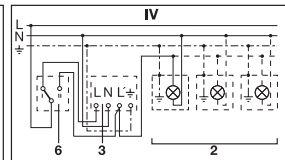
4. Připojení prostřednictvím přepínače pro trvalé osvětlení a automatický provoz Poloha I: automatický provoz Poloha II: ručně ovládané trvalé osvětlení Pozor: Vypnutí soustavy není možné, lze pouze přepínat mezi polohou I a polohou II.
