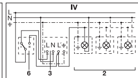
4. Ühendus rööpühendusega lülitiga pidevaks valgustuseks ja automaatujuhtimiseks Asend I: automaatrežiim Asend II: käsirežiim pidev valgustus Tähelepanu! Seadme väljalülitamine ei ole võimalik, valida saab ainult asendi I ja asendi II vahel.
